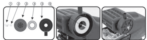
Fig. 2 – Conjunto del filtro
