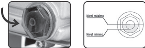
Fig. 4 – Nivel del aceite
